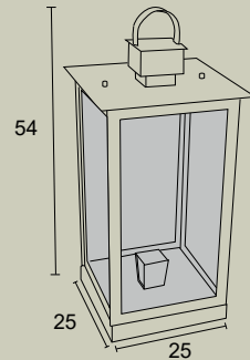
LA 431 IP54 – Indicado para uso externo 1x Alumínio e vidro transparente Medidas em cm
